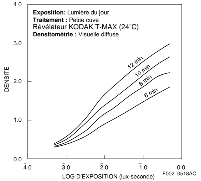
Courbes Caractéristiques
